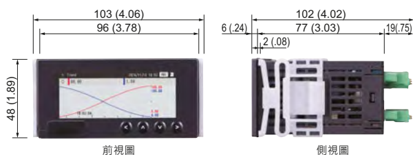
前視圖
