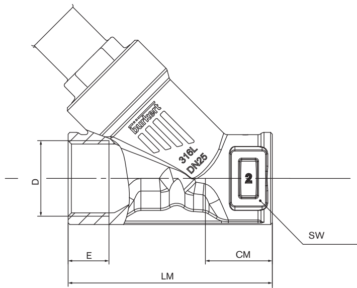
G, RC, NPT (EN ISO 228-1, ISO 7/1 /DIN EN 10226-2, ASME B 1.20.1)
